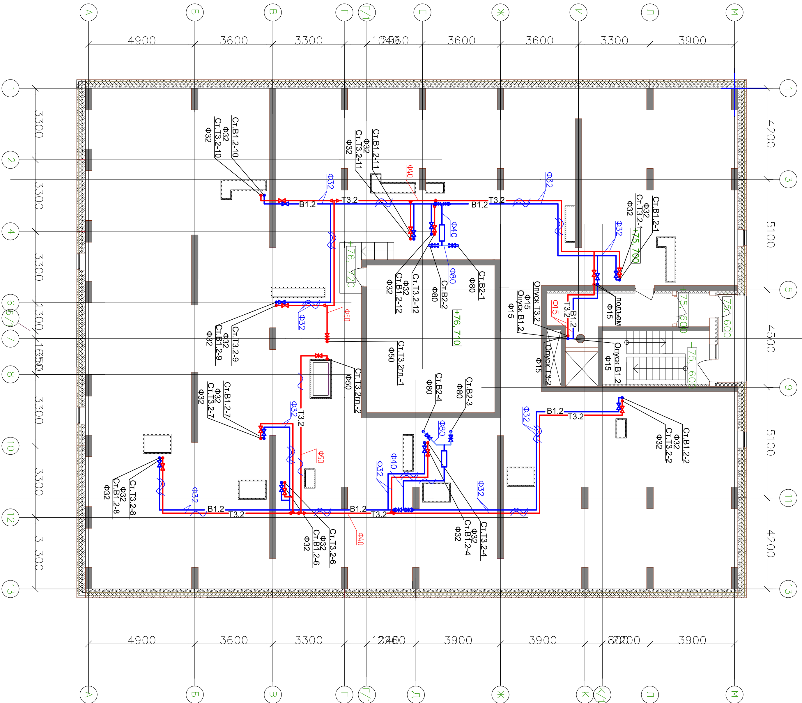
План технического этажа с сетями В1.2, В2, Т3.2
